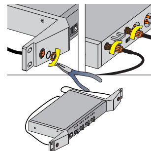
Figure 6: Monter l'antenne sur la façade avant
